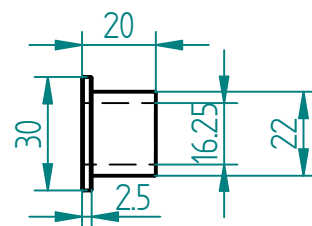
Optional T-bush Kit Part Number: TBush Kit 7/8 (ZP) 8 bolt
