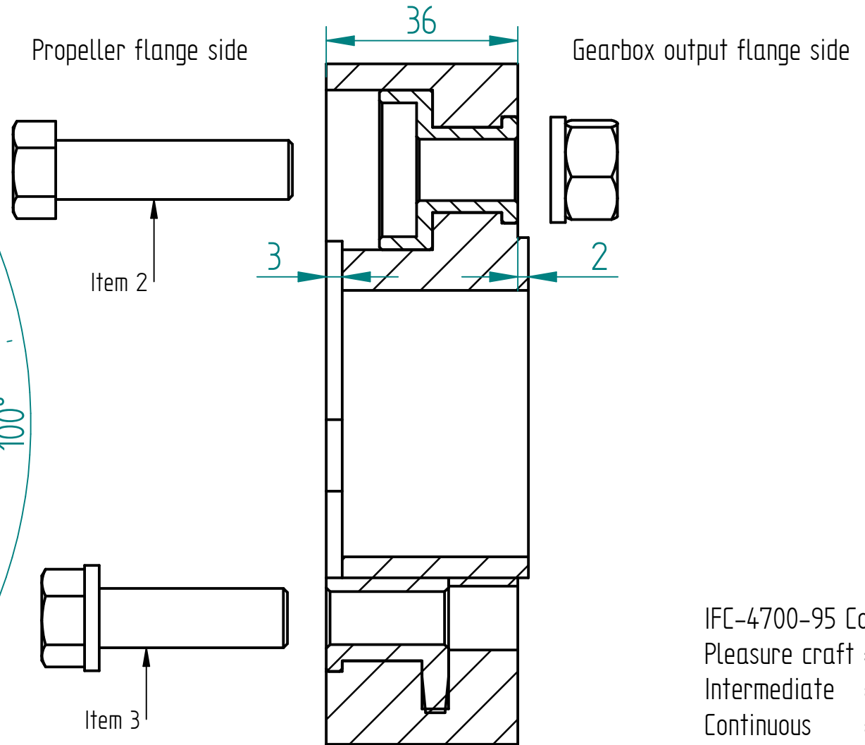
SECTION A-A
